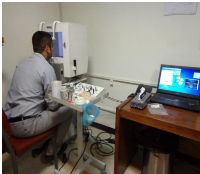
شکل ۱- دستگاه الکترواکولوگرافی دینامیک
